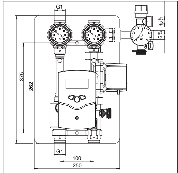
Maße „Regusol EL-130“ Station mit elektronischem Regler „Regtronic BS/2-B“
