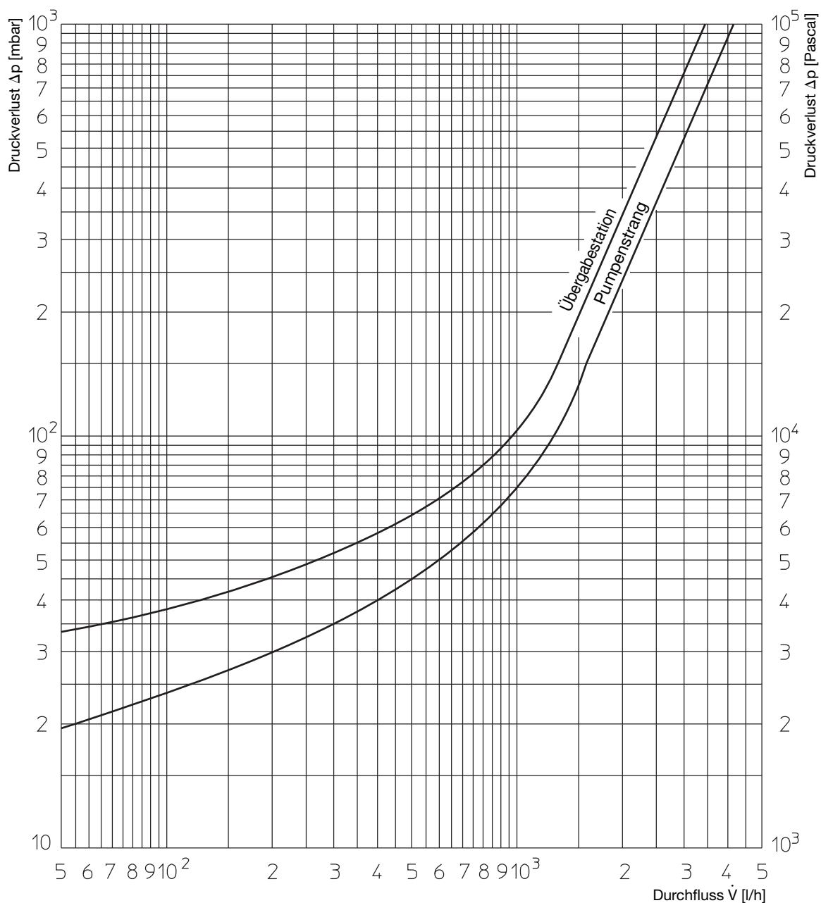
Durchflussdiagramm
