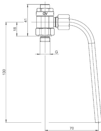
Réf. 4209102/4209103
