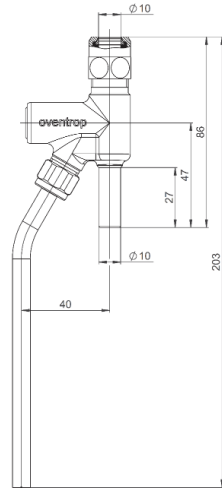
Réf. 4209202
