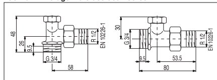
«Combi 2» filetage mâle des deux côtés
