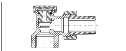
„Combi 2“ Eckform mit Innengewinde EN 10226-1
