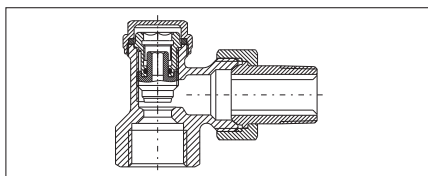
„Combi 3“ Eckform mit Innengewinde EN 10226-1
