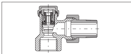
„Combi 4 und C“ Eckform mit Innengewinde EN 10226-1
