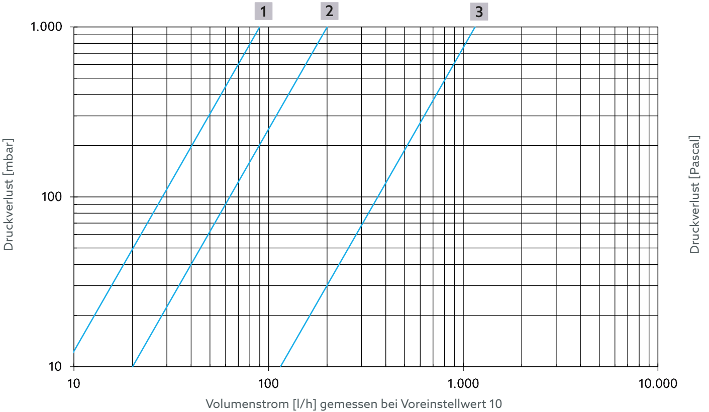
Abb. 17: Volumenstrom Thermische Regelung für Artikelnummer 4202504, 4202604, 4202704, 4202804
