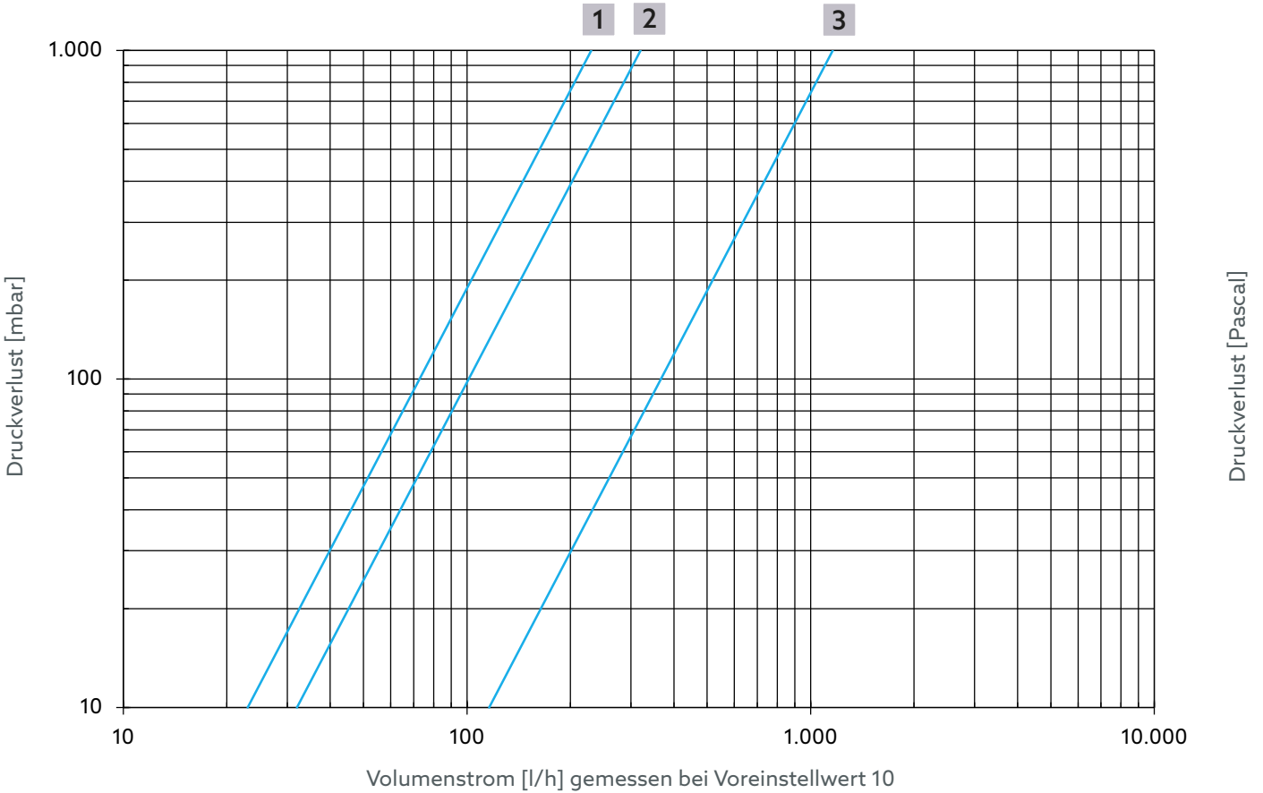
Abb. 18: Volumenstrom Thermische Regelung für Artikelnummer 4202553 und 4202753
