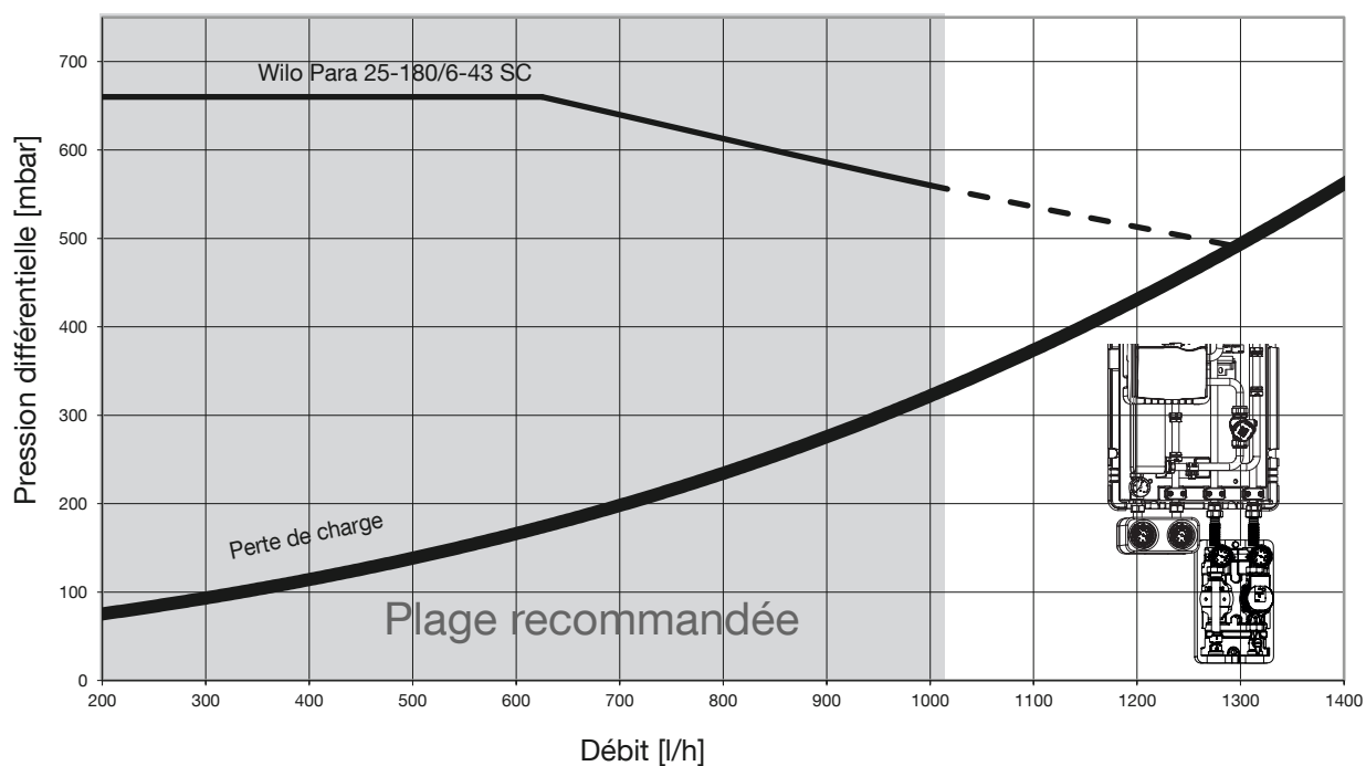
Fig. 5: Perte de charge circuit secondaire Regudis H-H
