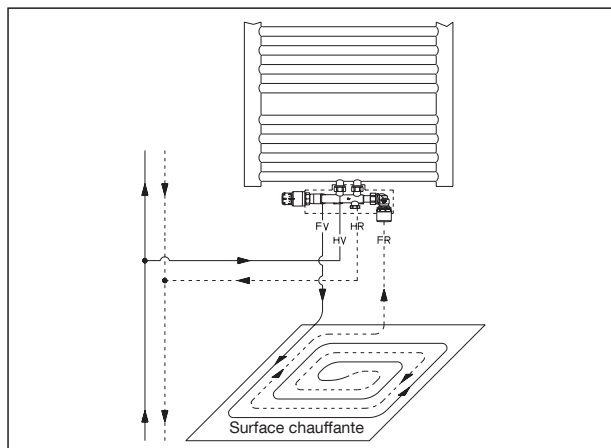
Schéma d'installation
