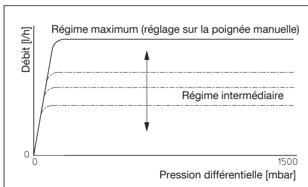
Courbes caractéristiques en régime intermédiaire
