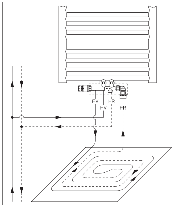
Schéma d'installation
