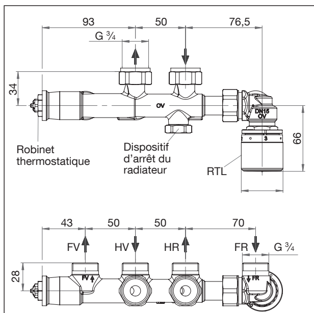
Encombres du raccord
