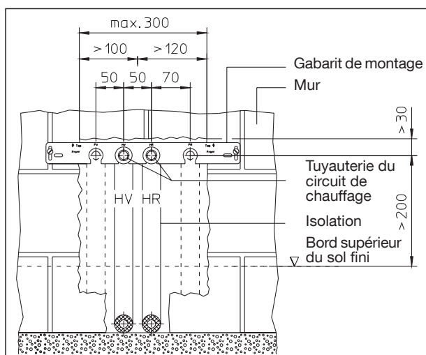
Vue frontale, raccordement circuit de chauffage
