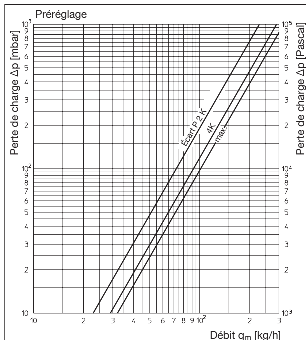
Diagramme de perte de charge, RTL (circuit de surface chauffante)
