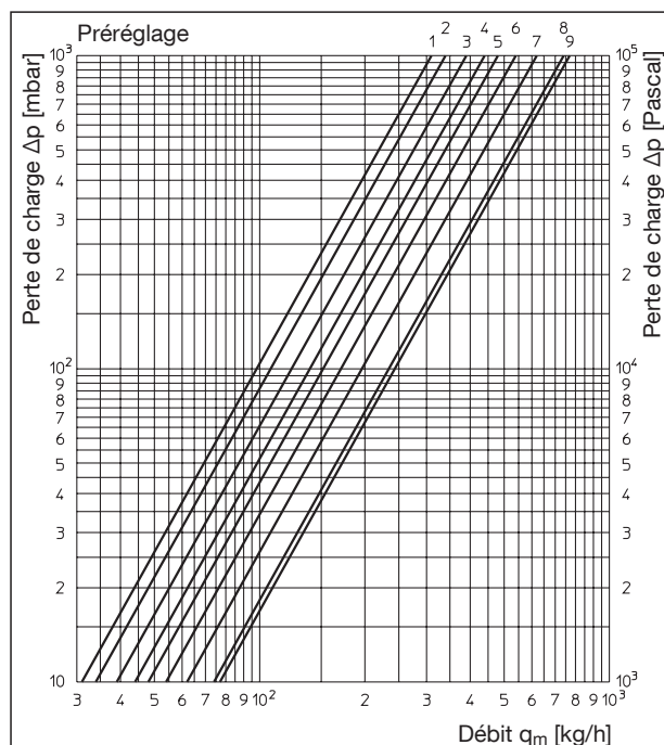
Diagramme de perte de charge, robinet thermostatique + RTL Robinet thermostatique pour un écart P de 2 K Limiteur de la température de retour pour un écart P de 2 K à 4 K Longueur de la tuyauterie : circuit surface chauffante 100 m Matériel de tube : tube multicouche « Copipe » 16 x 2 mm
