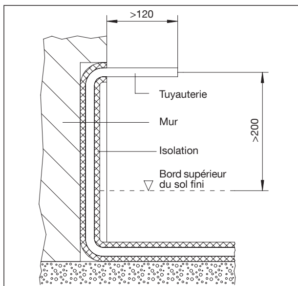
Vue en coupe, raccordement circuit de chauffage
