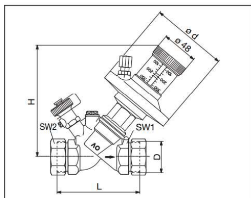
Typ regulátoru 10646/48 04-16 oboustranně vnější závit a převlečná matice
