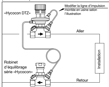
Illustr. 6.3: «Hycocan DTZ» Montage sur l'aller (seulement DN 32 + 40)
