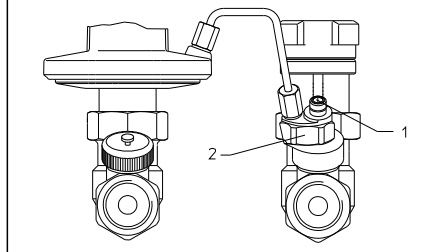
Illustr. 6.1: «Hycocan DTZ» Illustration du raccordement de la ligne d'impulsion, montage sur le retour
