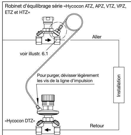
Illustr. 6.2: «Hycocan DTZ» Montage sur le retour
