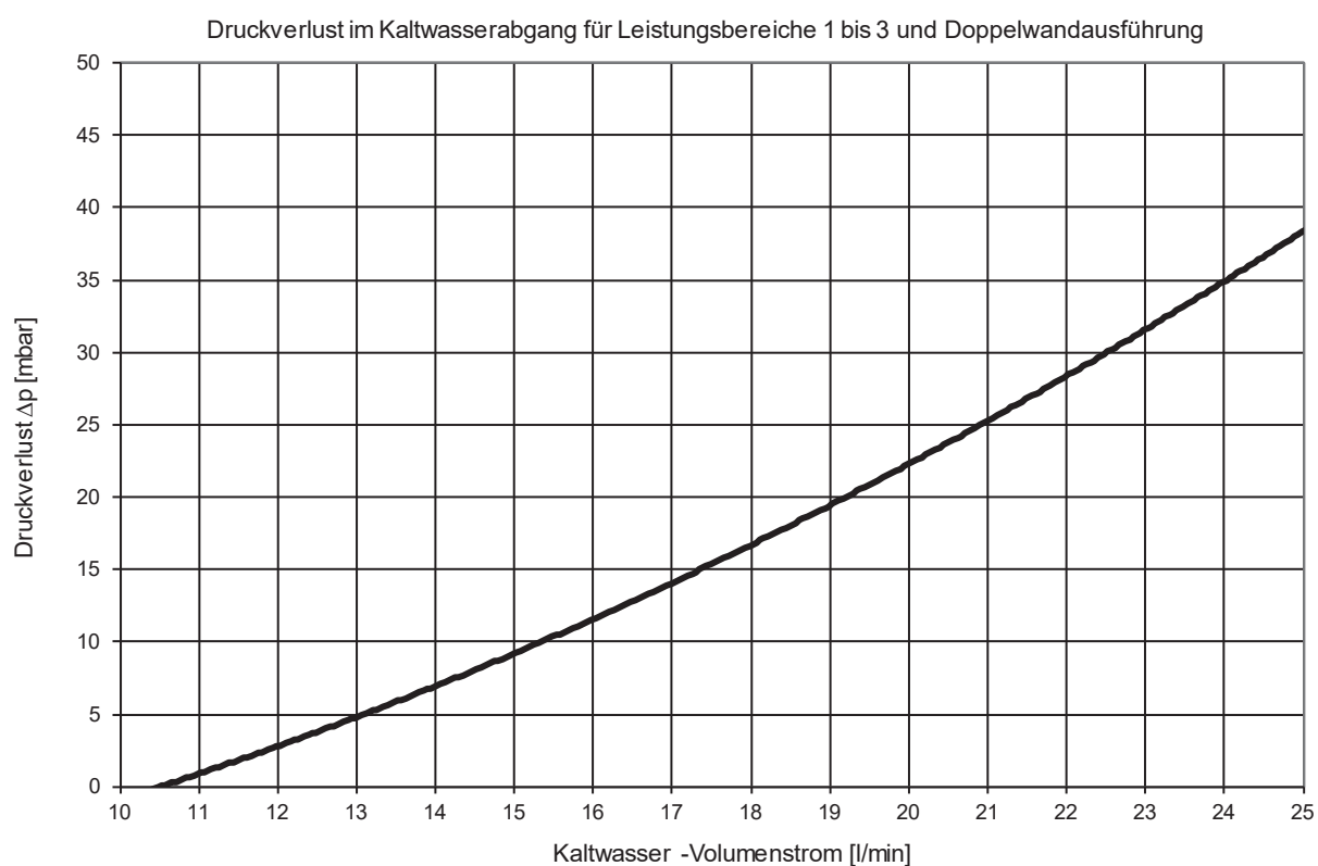
Abb. 50: Druckverlust im Kaltwasserabgang
