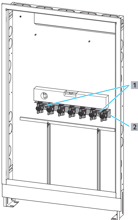
Abb. 13: Kugelhahn-Anschlusset montieren
