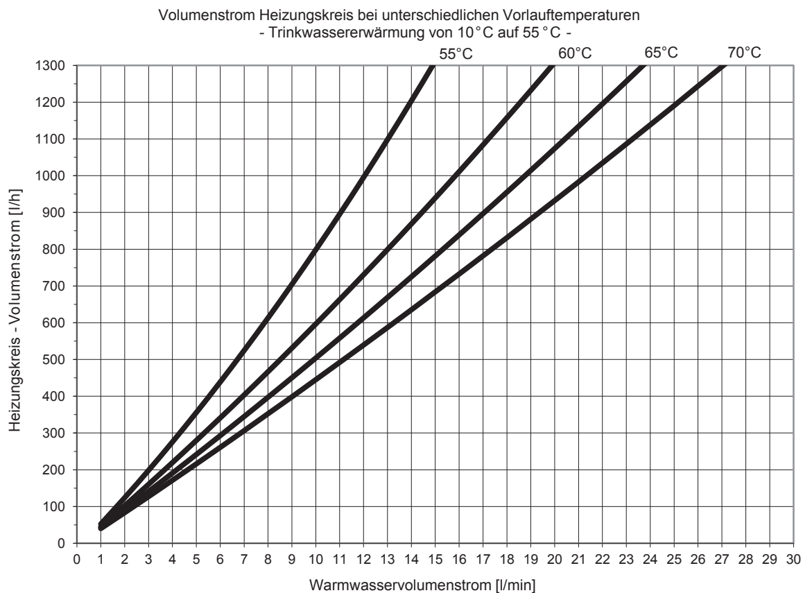
Abb. 63: Leistungsbereich 2, Trinkwassererwärmung auf 55 °C
