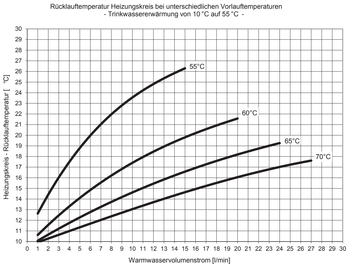
Abb. 64: Leistungsbereich 2, Trinkwassererwärmung auf 55 °C
