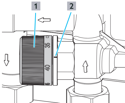
Abb. 33: Temperaturvorhalte-Regelset einstellen
