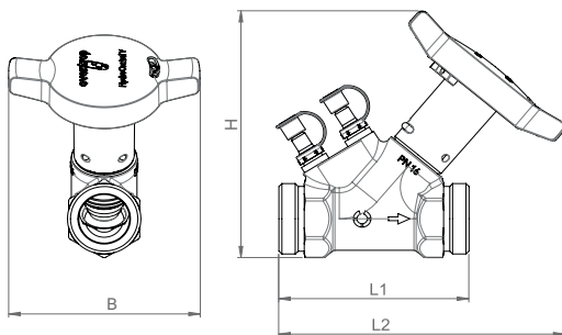
Fig. 3: Encombrenents vue de côté / vue de face - Version avec filetage mâle
