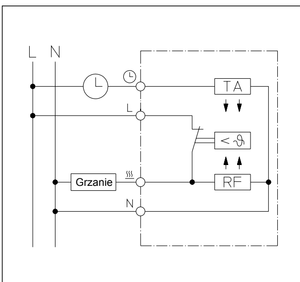
Schemat połączeń
