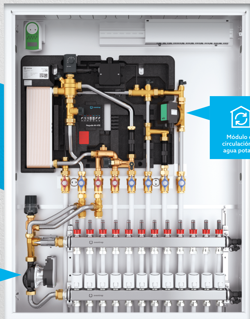
Módulo de control de temperatura de caudal
