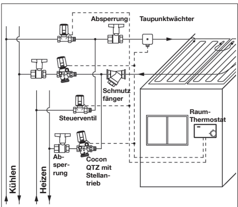
Abb. 7: Einbaubeispiel 2: Vielleitersystem
