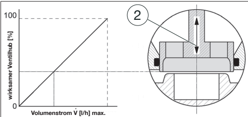
Abb. 5: Lineare Kennlinie der Reguliereinheit
