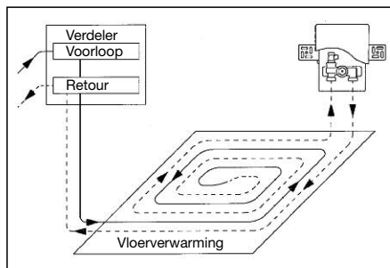
Inbouwplan
