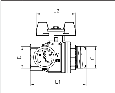
Fig. 6: Maße Kugelhahn
