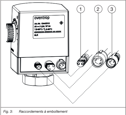
Fig. 3: Raccordements à emboîtement
