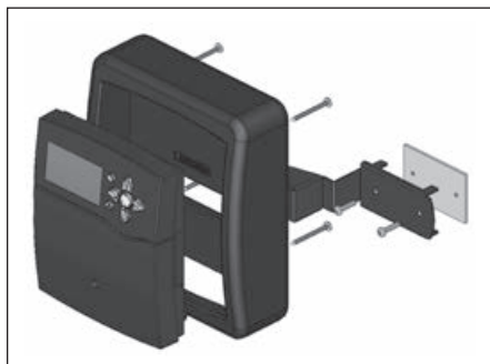
Fig. 1.1 Set ampliamento centralina per circuito di riscaldamento „Regumat-180“ DN 25 „nuovo“ con valvola a sfera per pompa
