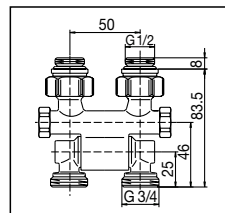
ZB-podwójne przyłącze z odcieciami, kątowno-proste (dowolny kąt podejścia) \frac{3}{4} " ( \frac{3}{4} " NZ x \frac{3}{4} " GZ)
