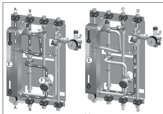
Primärseite Sekundärseite (Beispielhaft Anschluss zum Rohrnetz von oben)
