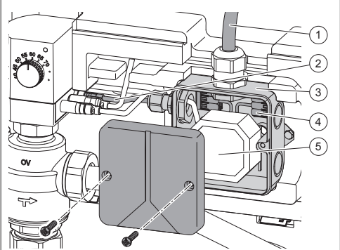
Abb. 1: Aufbau
