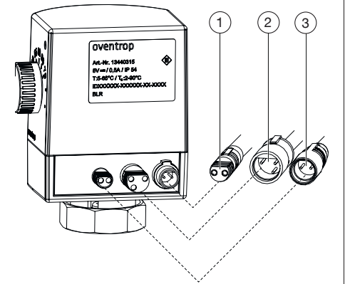
Abb. 3: Steckverbindungen
