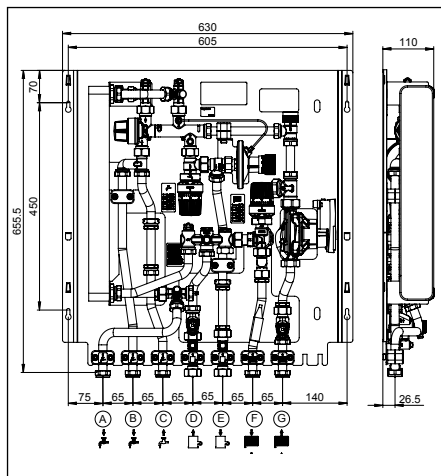
Abb. 4.4 Abmessungen mit gemischtem Heizkreis
