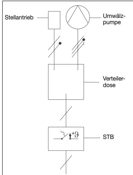
Abb. 4.1 Systemdarstellung Verkabelung
