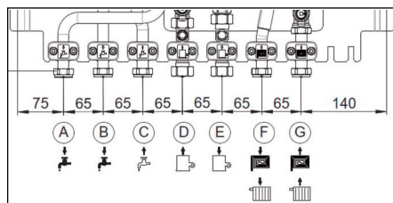
Fig. 4.3 Dimensioni collegamenti
