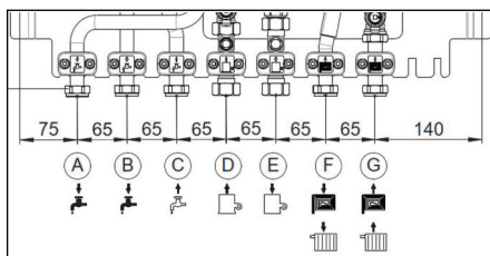
Abb. 4.3 Anschlussmaße
