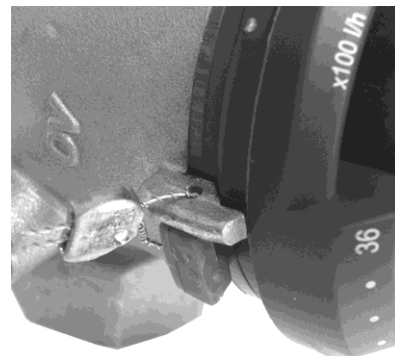
Abb. 26: Einstellung des max. Volumenstroms am „Cocon QTZ“
