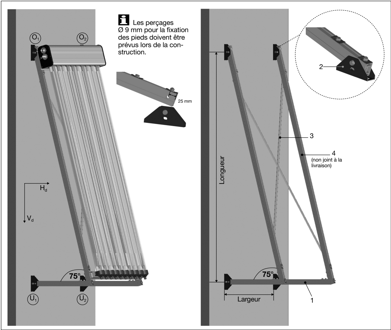
OKP-Montage sur châssis libre réf. 136 12 78 (Capteurs et profilé de cadre pos. 4 non joints à la livraison)
