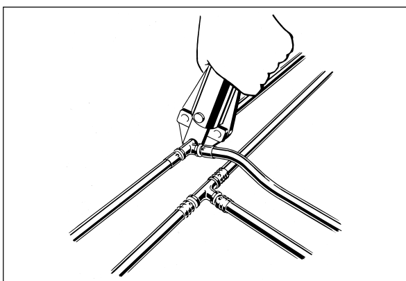
Realizarea îmbinărilor
