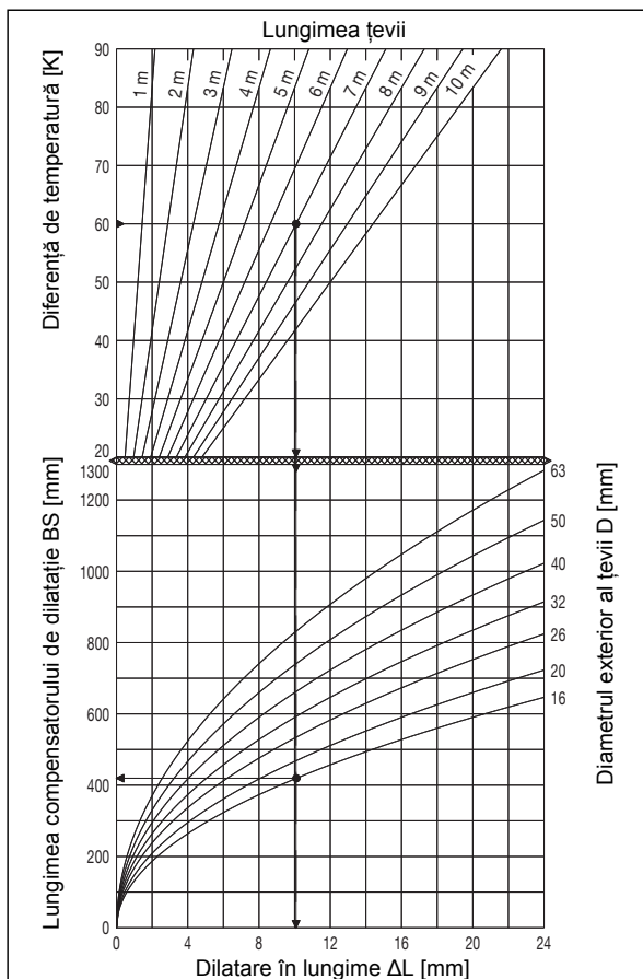
13 Diagramă pentru țeava multistrat „Copipe“ de la Oventrop:
