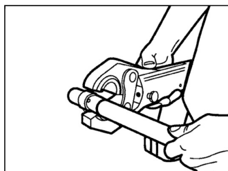
Aplicarea cleștelui de presare (50 mm)
