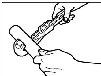
Tăierea perpendicular pe axa țevii
