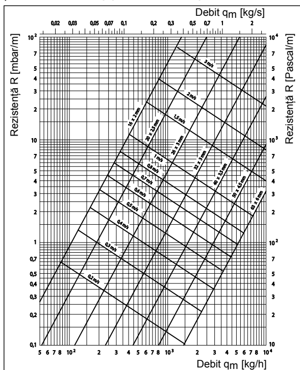
13 Diagramă pentru țeava multistrat „Copipe“ de la Oventrop:
