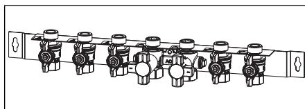
Abb. 1.1 Kugelhahnanschlussleiste
