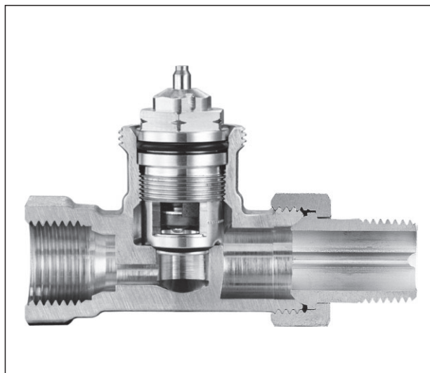
Проходной вентиль серии „AV 9“
