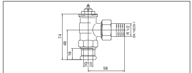
Угловой вентиль
