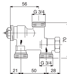
Вентиль „ТКМ“ (для однотрубных/двухтрубных систем)
