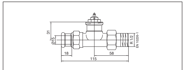
Прходной вентиль
