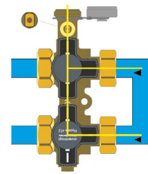
Изолиране и източване от страна на уреда
