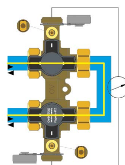
Измерване на диференциалното налягане, напр. с OV-DMC 3
