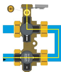
Пълнене и промиване от страна на уреда
