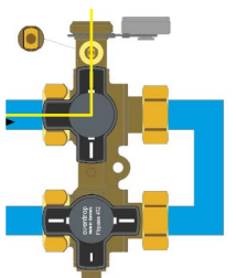
Източване, обезвъздушаване и промиване от страна на инсталацията
