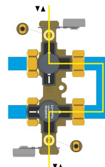
Допълване, обезвъздушаване и промиване от страна на уреда с втори сферичен вентил за пълнене и източване
