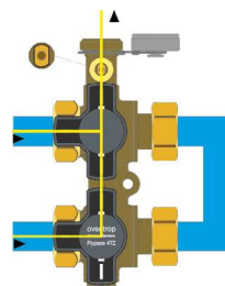
Пълнене и обезвъздушаване от страна на инсталацията
