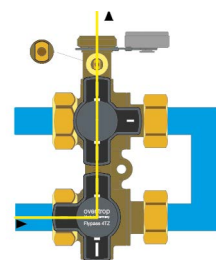
Източване от страна на инсталацията/уреда, обезвъздушаване и промиване от страна на инсталацията
