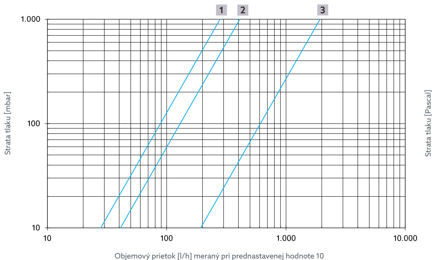
Obr. 19: Objemový prietok termoregulácie pre číslo položky 4202506, 4202606, 4202706, 4202806
