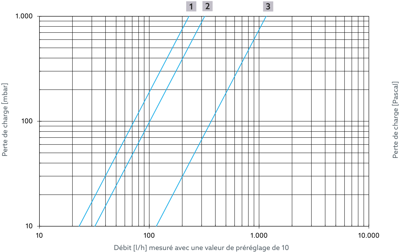
Fig. 18: Débit du réglage thermique pour réf. 4202553 et 4202753
