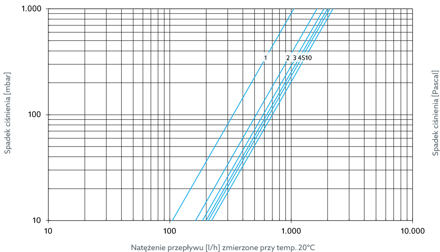
Ryc. 16: Nastawa domyślna natężenia przepływu DN 20
