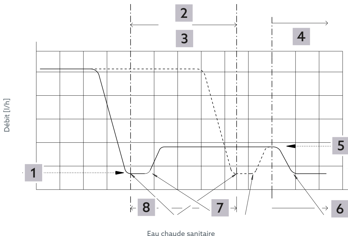
Fig. 6: Comportement de régulation thermique
