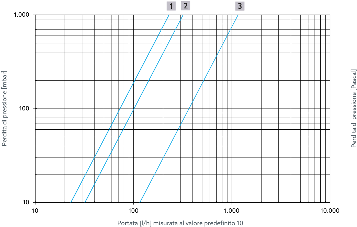
Fig. 18 - Portata regolazione termica dei codici articolo 4202553 e 4202753
