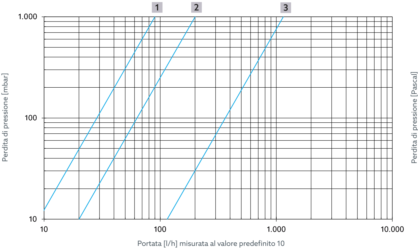
Fig. 17 - Portata regolazione termica dei codici articolo 4202504, 4202604, 4202704, 4202804
