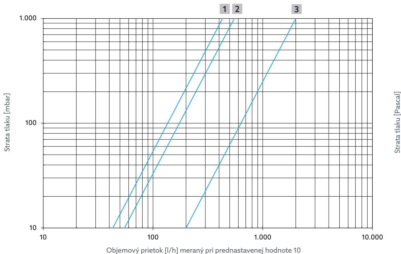
Obr. 20: Objemový prietok termoregulácie pre číslo položky 4202554 a 4202754
