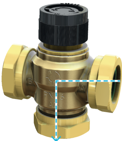
Рис. 2: Канал А–АВ
