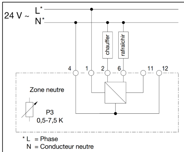
Schéma électrique
