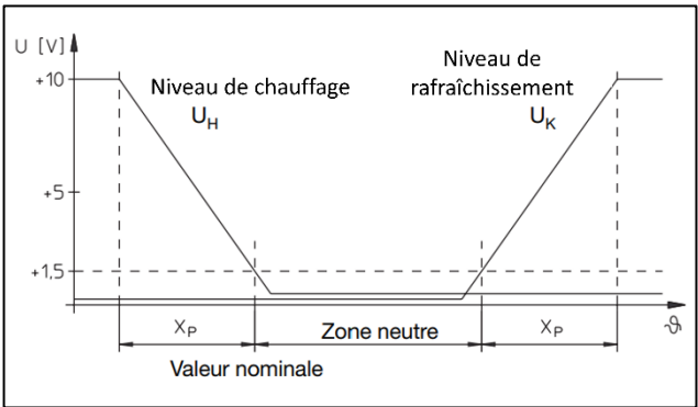
Diagramme fonctionnel
