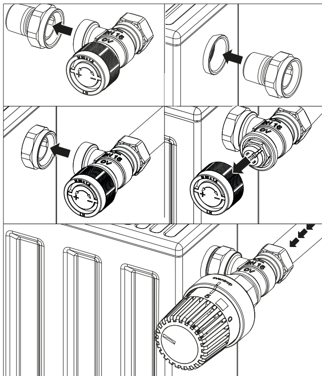
Abb. 2: Montagebeispiel Thermostatventil
