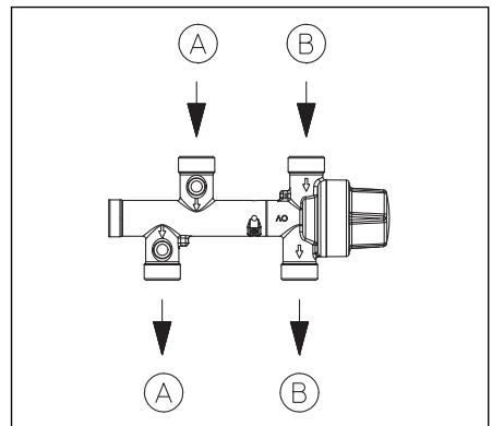
Abb. 5.4: Proportional-Mengenregler
