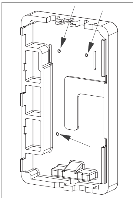
Fig. 6.2: Partie arrière de la coquille d'isolation, gabarit de perçage
