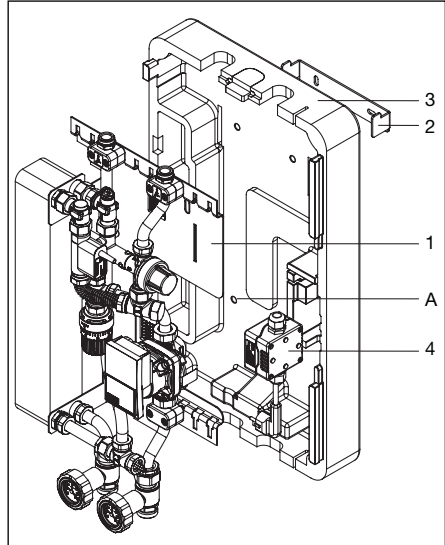
Abb. 6.3: Wandbefestigung
