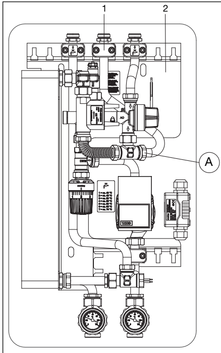
Abb. 6.4: Zirkulationsleitung anschließen
