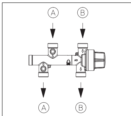
Fig. 5.4: Robinet pressostatique à priorité E.C.S.
