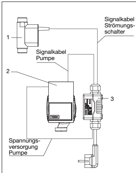
Abb. 5.5: Elektronikkomponenten
