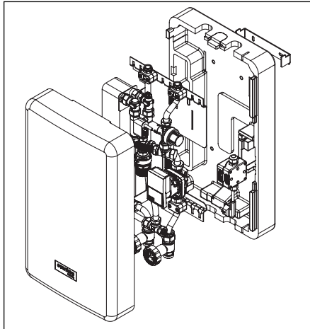
Abb. 5.1: Gesamtansicht Armaturenbaugruppe
