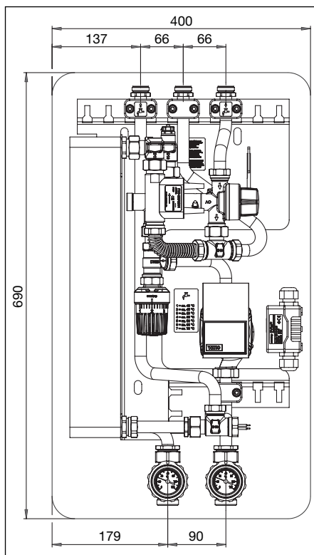
Fig. 6.1: Montage, indications en mm
