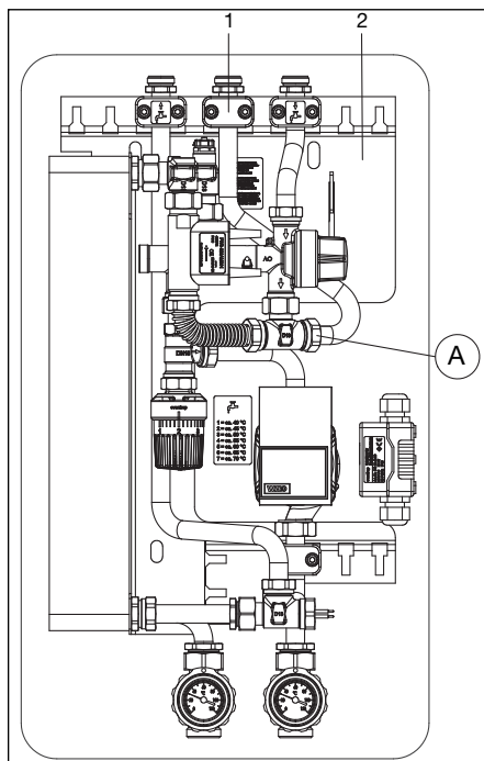
Fig. 6.4: Raccordement des conduites d'alimentation
