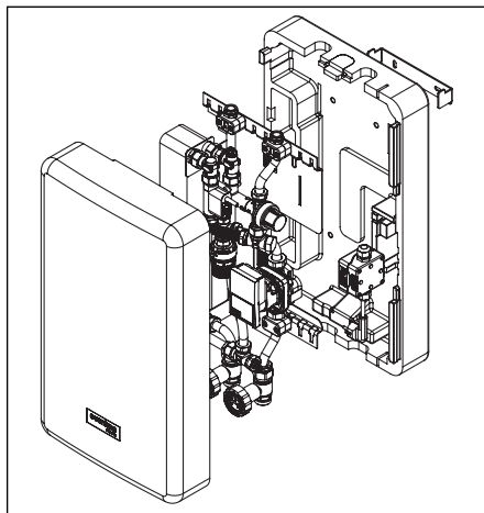
Fig. 5.1: Vue d'ensemble groupe de robinetterie
