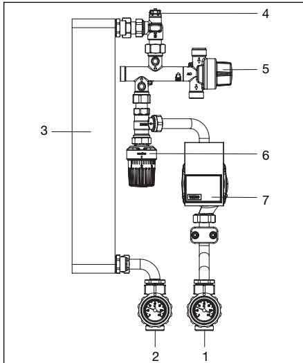
Abb. 5.2: Primärkreislauf
