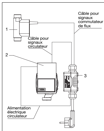
Fig. 5.5: Composants électroniques
