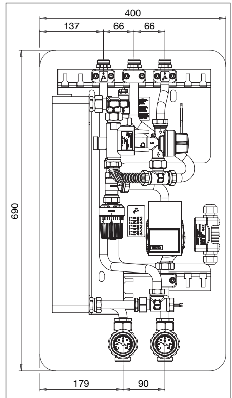
Abb. 6.1: Montage, Angaben in mm
