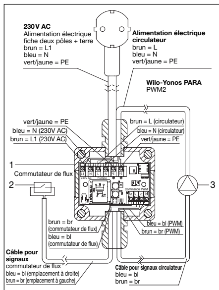
Fig. 6.6: Câblage du circuit primaire
