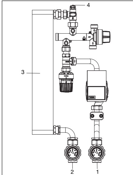
Abb. 7.1: Entlüften „Regumaq XH“
