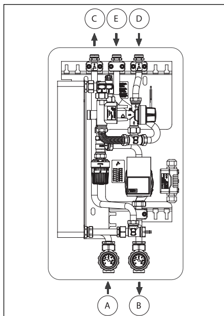
Fig. 6.5: Raccordement des conduites d'alimentation
