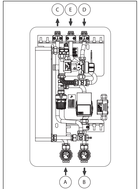
Abb. 6.5: Versorgungsleitungen anschließen
