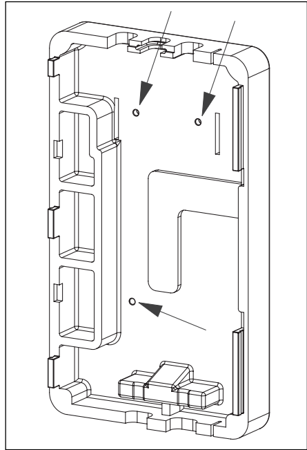
Abb. 6.2: Unterschale, Bohrschablone
