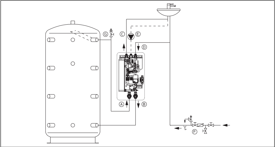
Abb. 5.6: Systemdarstellung
