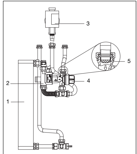
Abb. 5.3: Sekundärkreislauf
