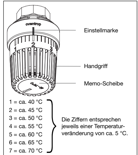
Abb. 7.2 Temperaturregler
