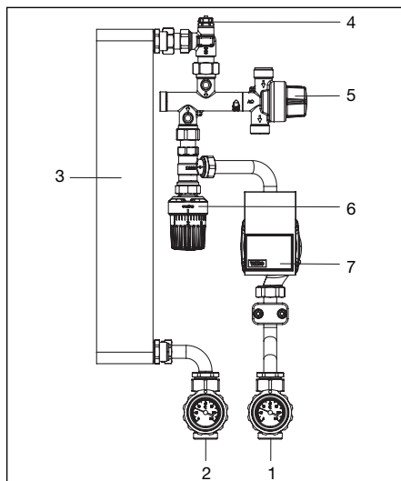
Fig. 5.2: Circuit primaire
