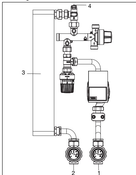
Fig. 7.1: Purge «Regumaq XH»
