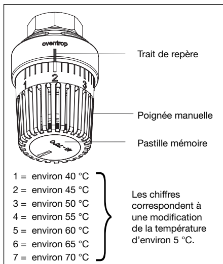
Fig. 7.2: Régulateur de température
