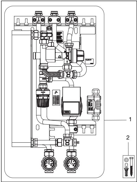
Abb. 3.1 Lieferumfang
