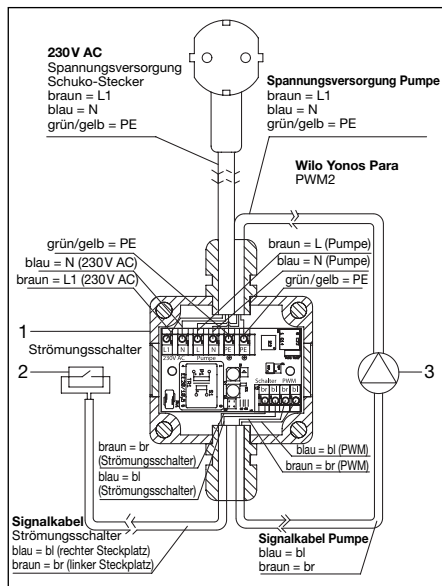
Abb. 6.6: Verkabelung Primärkreis
