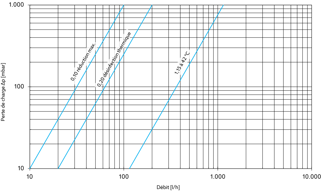
Débit réglage thermique Aquastrom T DN 15
