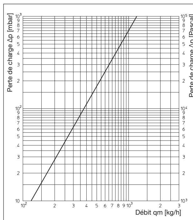
Raccords d'arrêt ZB, orientables Réf. 1015711/81
