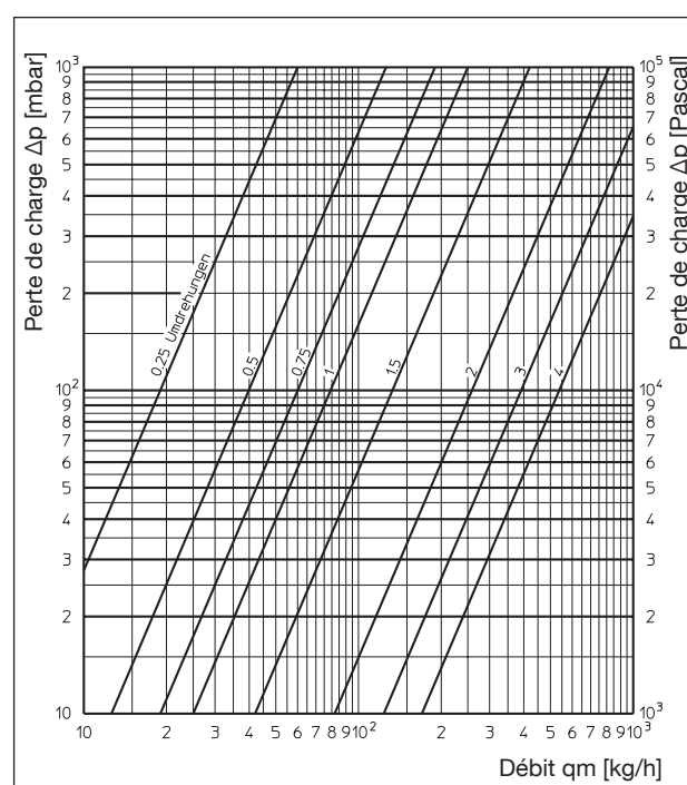
Raccords ZBU et raccords seuls en service bitube
