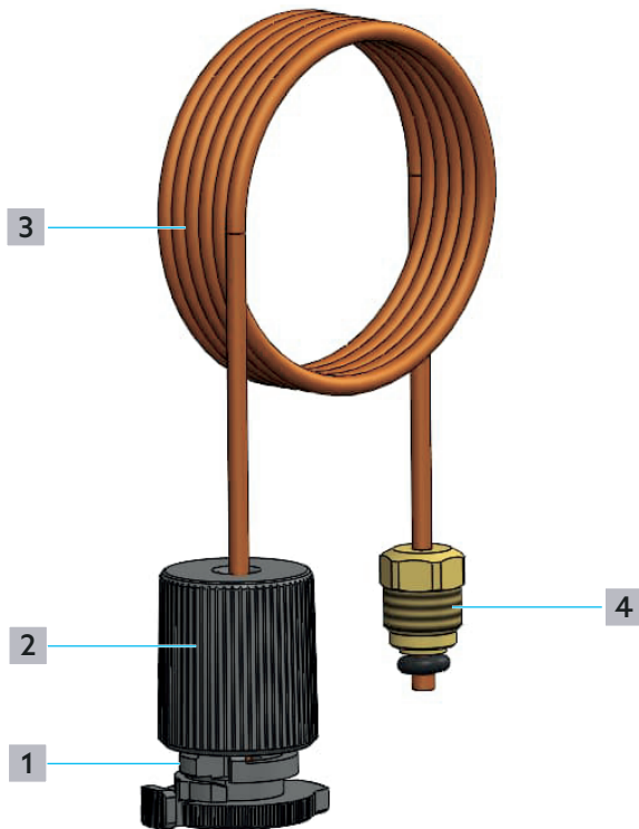
Afb. 4: Opbouw pulsleiding
