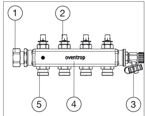
Abb. 1: Aufbau Vorlauf
