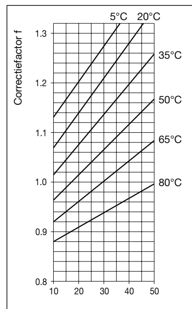
Gewichtsaaendeel propyleenglycol [%]
