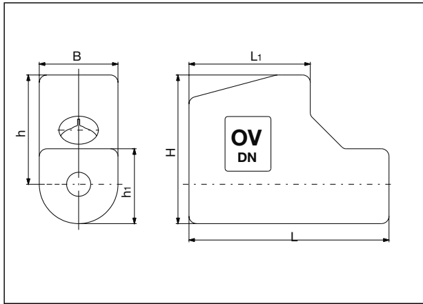
Isolatieschalen
