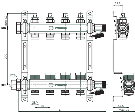
Fig. 6: Abmessungen
