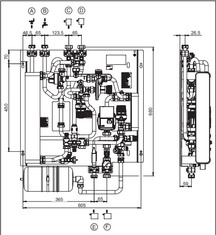
Fig. 2 Encombres
