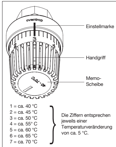
Abb. 4 Einstellung Trinkwassertemperatur
