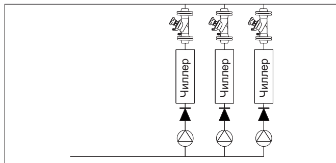
Пример: Система охлаждения с фланцевыми регулируемыми вентилем
