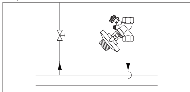
Пример: Регулирование расхода, например, в системе охлаждения. Преднастройка на регуляторе легко считывается.
