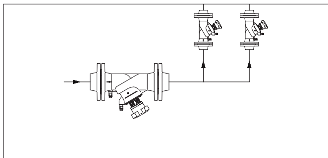
Пример: Система центрального отопления с фланцевыми регулируемыми вентилем
