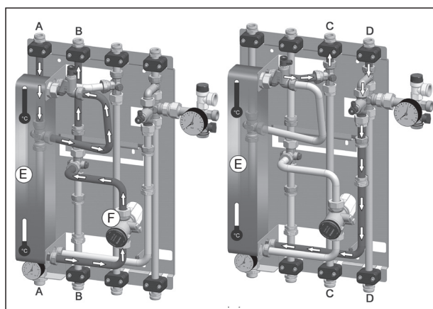
Côté primaire Côté secondaire (Exemple de raccordement par le haut au réseau de tuyauterie)
