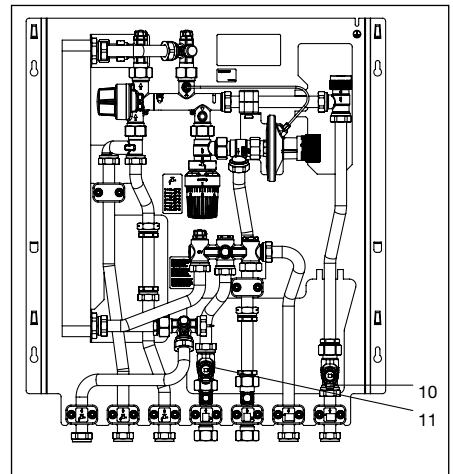
Abb. 8.1 Einbauposition Schmutzfänger
