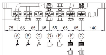
Fig. 4.3 Dimensioni collegamenti
