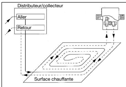
Croquis d'installation
