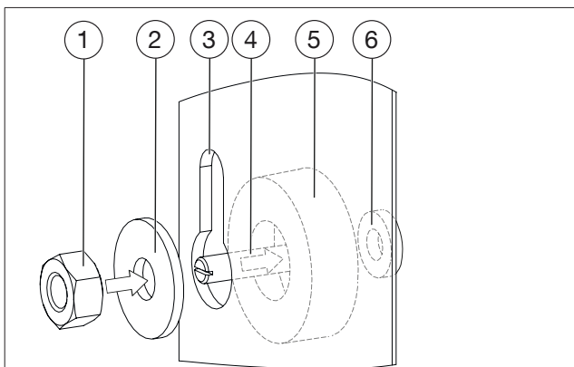
Abb. 5: Montage Befestigungspunkte „Regudis W-HTU“
