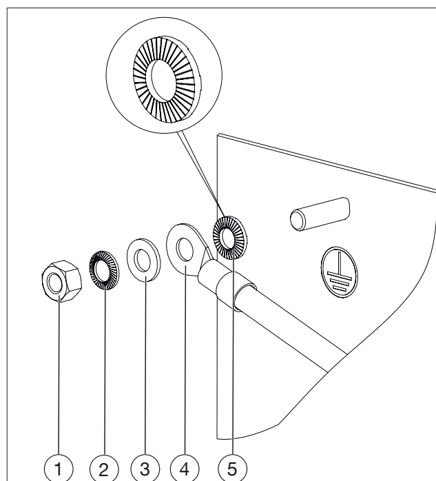
Fig. 9: Configuration du point central de mise à la terre
