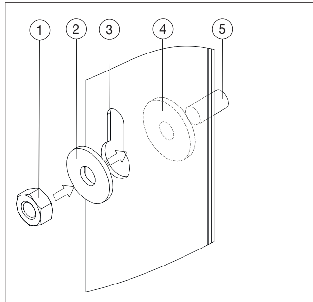
Abb. 6: Montage Befestigungspunkte „Regudis W-HTF“
