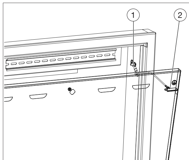
Fig. 8: Mise à la terre de la porte
