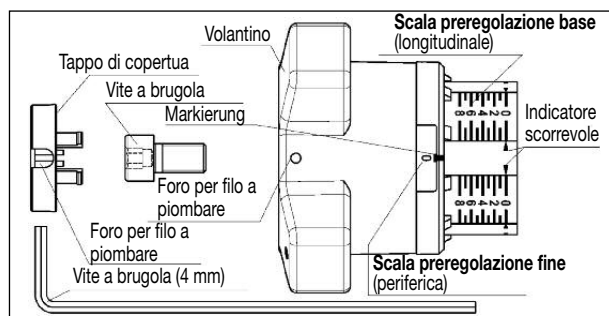
Fig. 7.1 Prerregolazione
