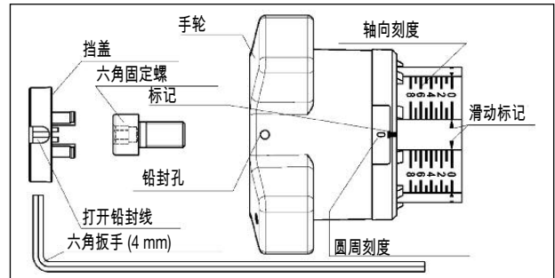
图 7.1 预设
