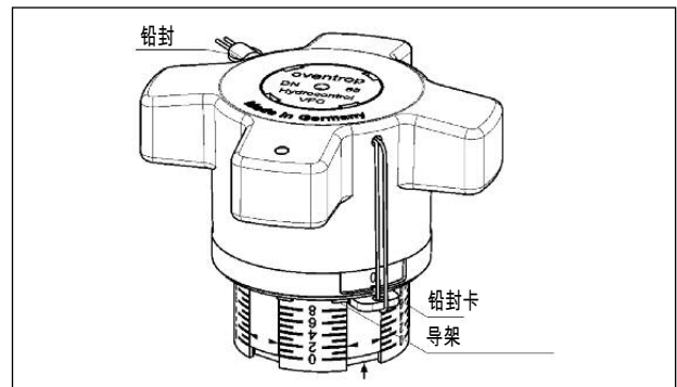
图7.2 手轮的锁定
