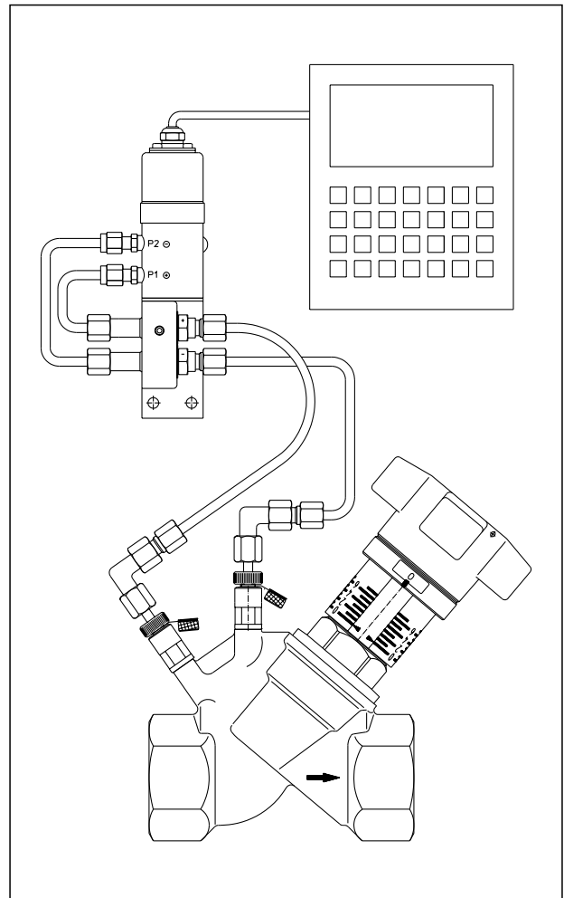
Exemple d'installation capteur de mesure de la pression différentielle
