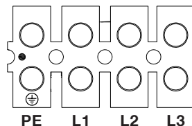
Abb. 6: Anschlussklemmen
