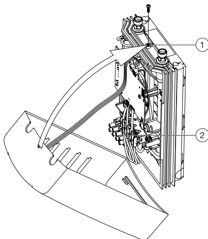
Abb. 5: Durchlauferhitzer öffnen
