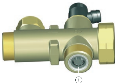
Abb. 4: Volumenstrombegrenzer
