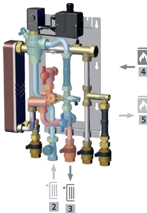
Fig. 3: Mode chauffage
