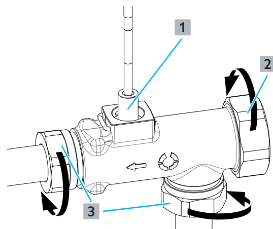
Fig. 24: Montage du capteur de débit
