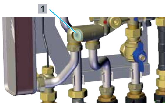
Fig. 25: Nettoyage de l'élément filtrant
