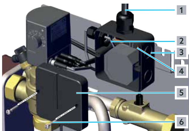
Fig. 13: Branchement électrique de la station d'appartement
