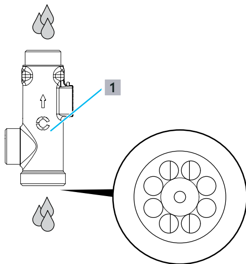
Fig. 23: Nettoyage du capteur de débit sous l'eau courante
