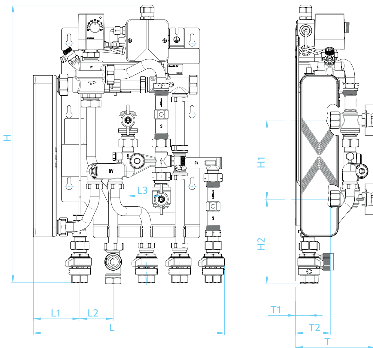
Fig. 6: Encombrements
