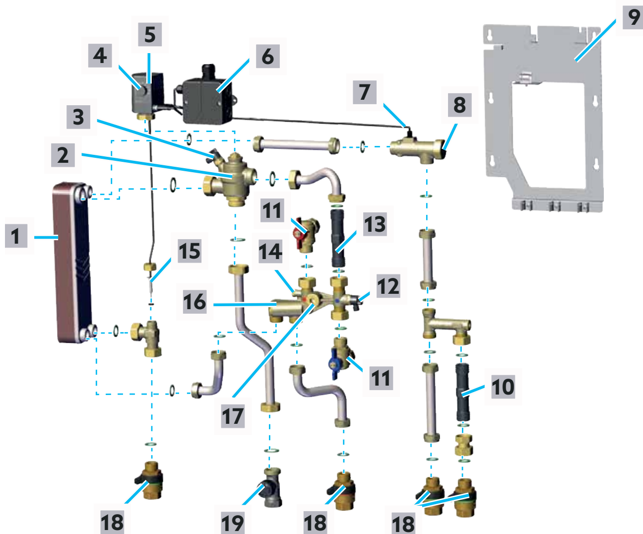
Fig. 2: Vue d'ensemble de la station d'appartement Regudis W-CE
