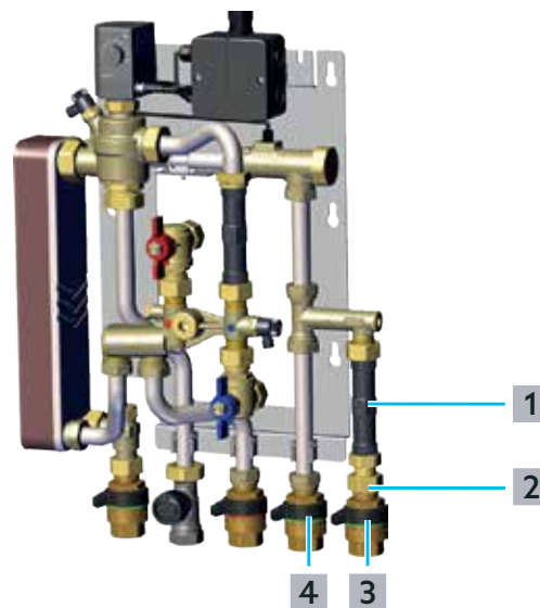
Fig. 11: Montage du compteur d'eau
