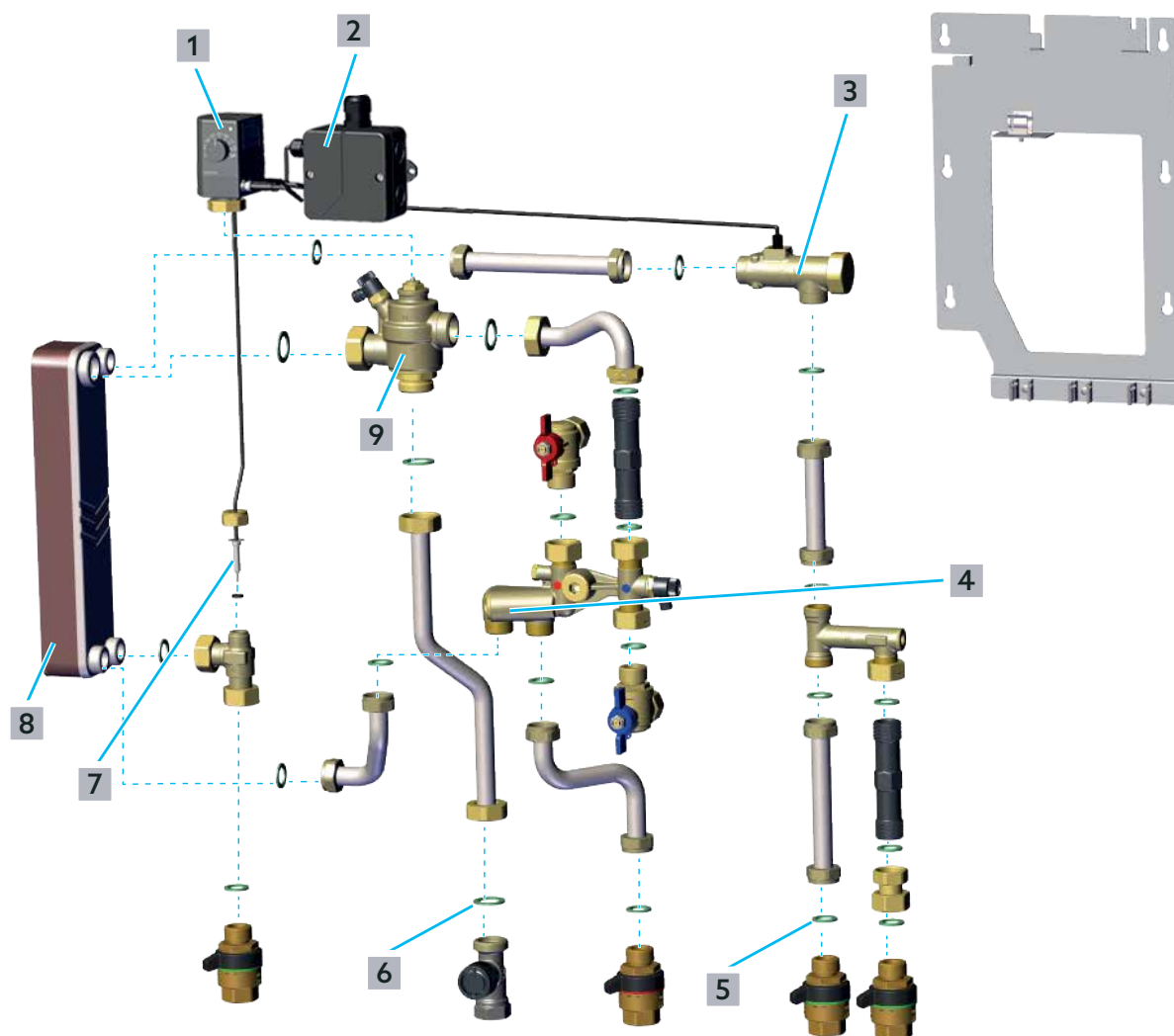
Fig. 8: Pièces de rechange
