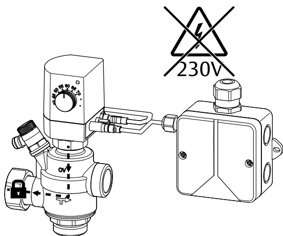
Fig. 1: Le robinet de régulation se ferme en cas de coupure de courant
