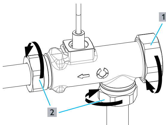
Fig. 22: Démontage du capteur de débit
