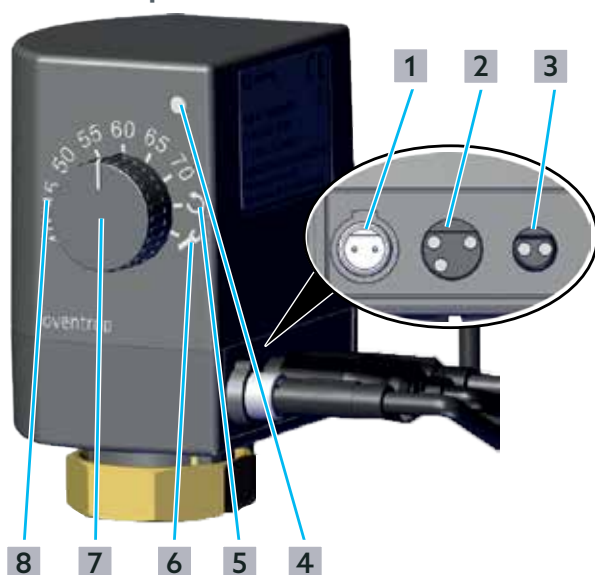
Fig. 5: Moteur avec régulation intégrée de la température E.C.S.
