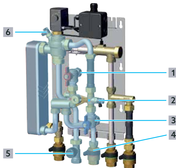
Fig. 14: Remplissage et purge du circuit de chauffage
