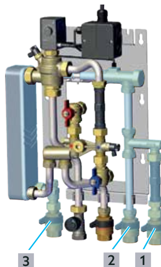
Fig. 15: Remplissage du circuit E.C.S.
