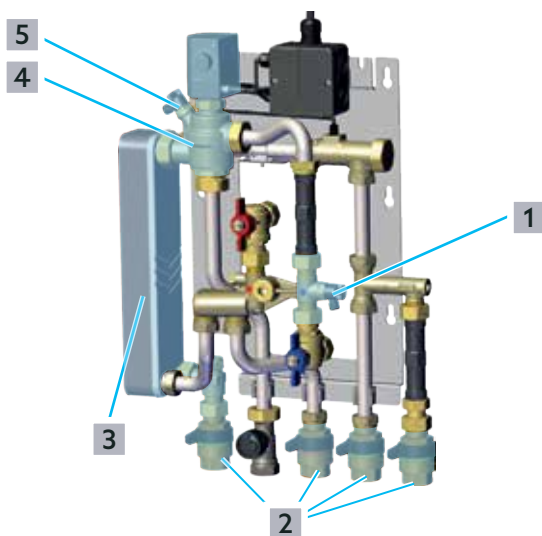
Fig. 19: Démontage et nettoyage de l'échangeur de chaleur
