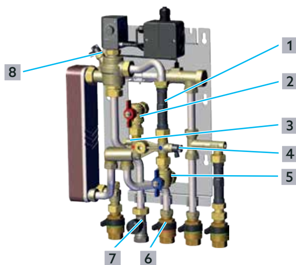
Fig. 10: Montage du compteur de calories
