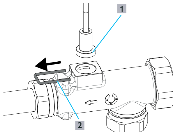
Fig. 21: Desserrage de l'agrafe de sécurité
