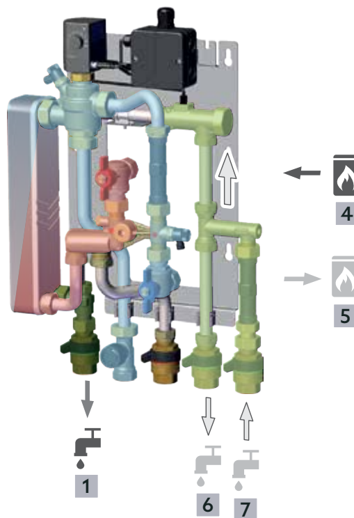
Fig. 4: Mode E.C.S.
