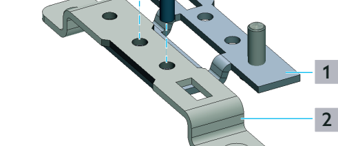
1 Dispositif de compensation de montage pour distributeurs/collecteurs pour circuits de chauffage Multidis
